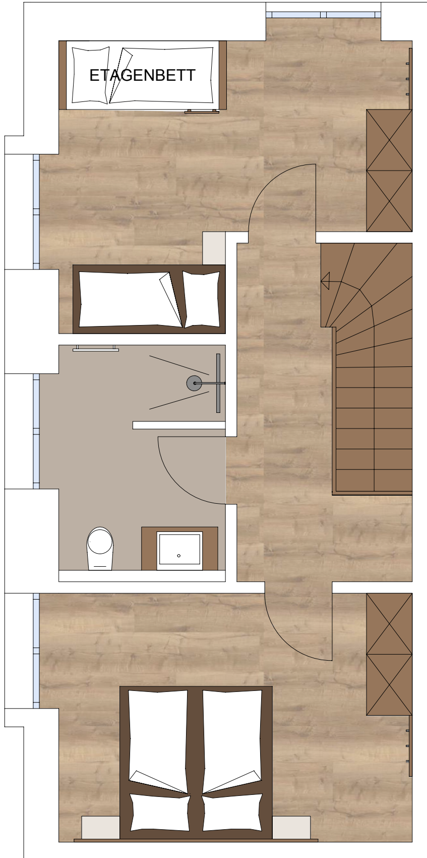
GRUNDRISS OBERGESCHOSS
