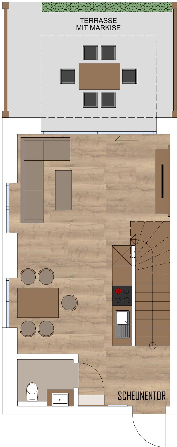
GRUNDRISS ERDGESCHOSS
